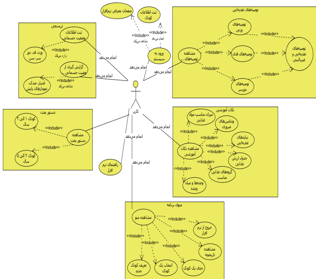
نمودار ۲: نمودار مورد کاربری
