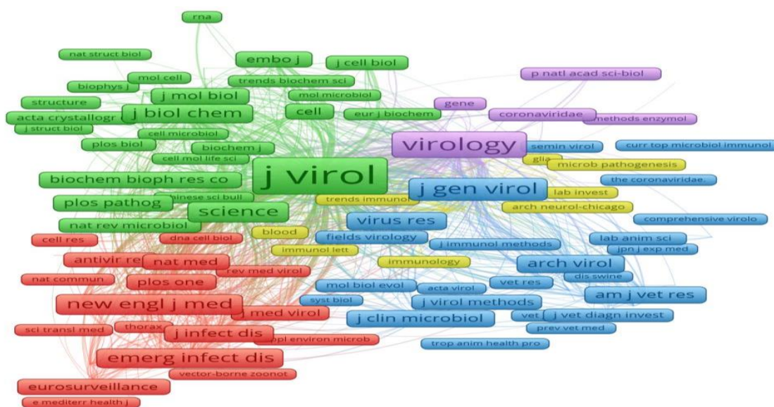
شکل ۴: شبکه هم‌استنادی مجلات برجسته موزه‌ی کرونا ویروس دارای حداقل فراوانی ۵۰
