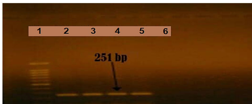
شکل ۳: PCR ژن CTX با اندازه ی ۲۵۱ bp. چاهک ۱: مارکر ۱۰۰-bp، چاهک ۲: کنترل مثبت، چاهک های ۳، ۴، ۵: جدایه های مثبت، چاهک ۶: کنترل منفی
