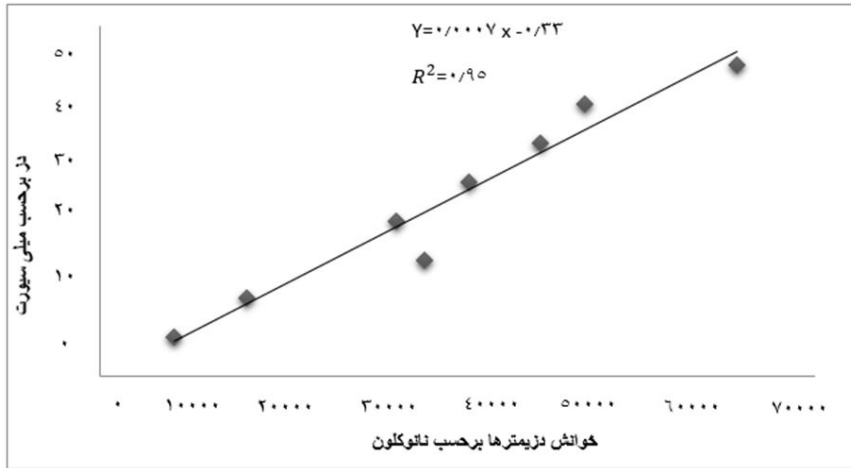
شکل ۱: منمنی دز در مقابل خوایش دزیمترها که با استفاده از کالیبراسیون RCF به دست آمد
