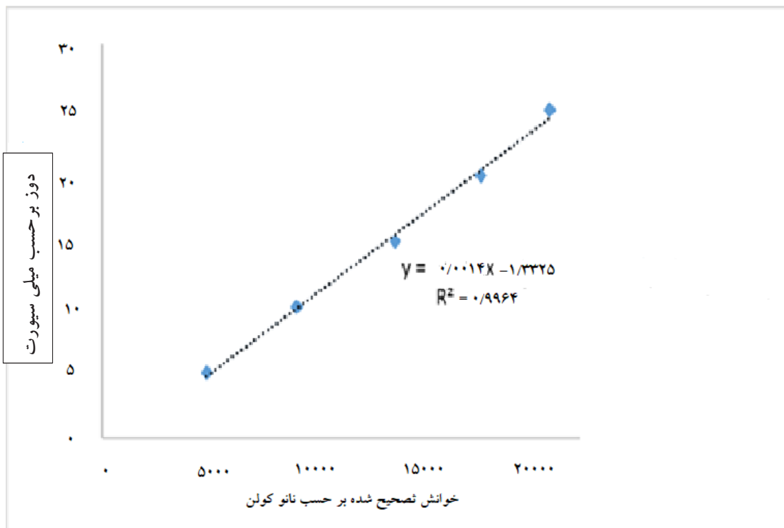
نمودار ۱: منمنی کالیبراسیون دوزیمترهای TLD
